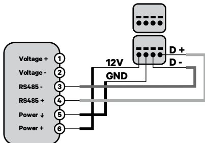
SPM1-100-AC
